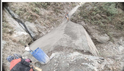
छरछरेमा कज वे निर्माण
